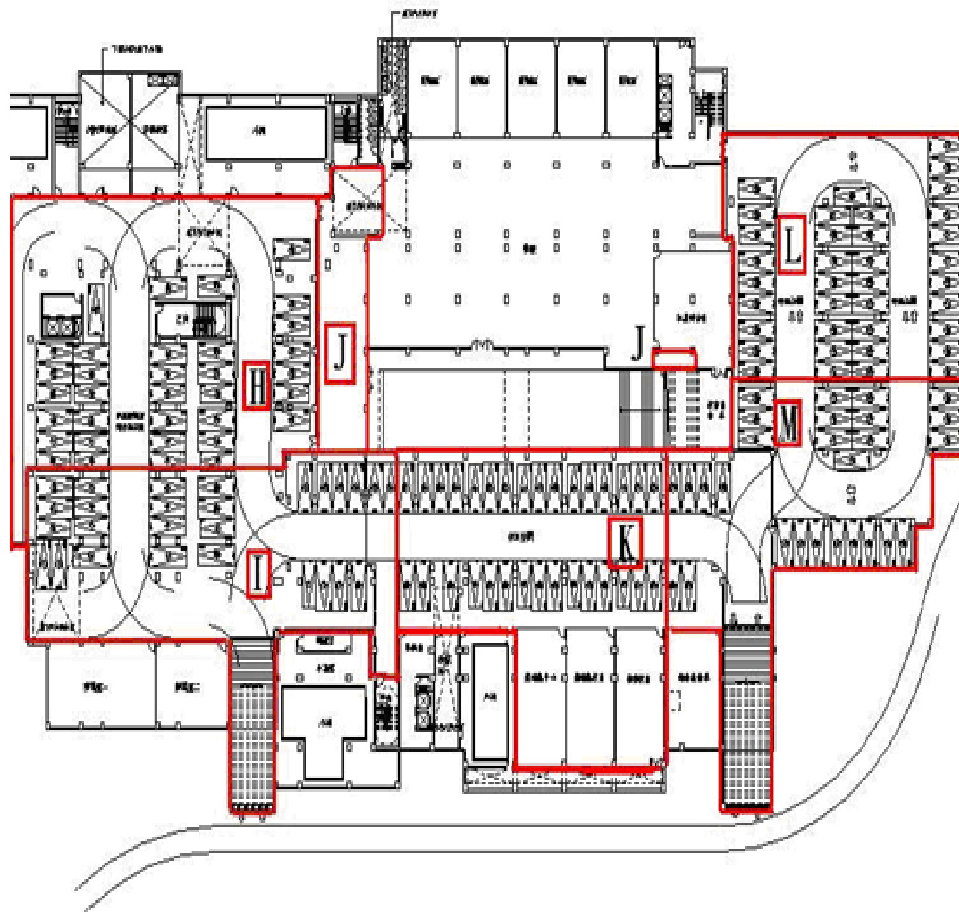
新生醫專地下室平面圖
